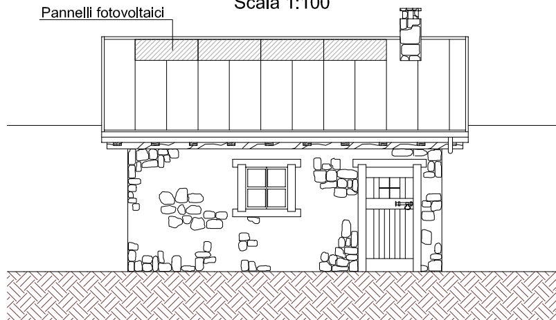
PROSPETTO TIPO Scala 1:100
