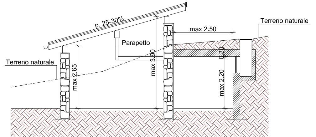
SEZIONE TIPO Scala 1:100
