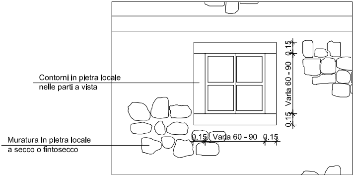
PARTICOLARE FINESTRA CON CONTORNI IN PIETRA Scala 1:50
