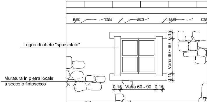
PARTICOLARE FINESTRA CON CONTORNI IN LEGNO Scala 1:50
